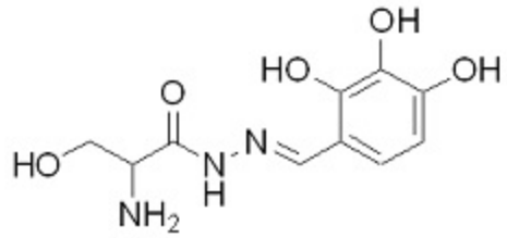
PC-3580601, DMSO-d6
